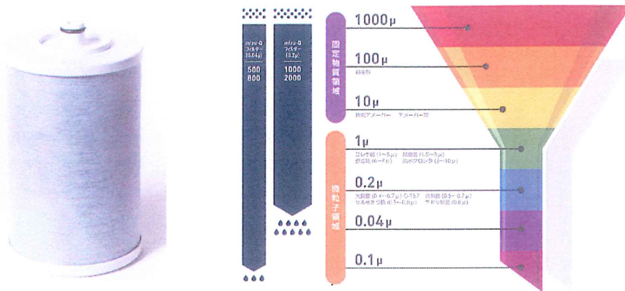
mizu-Qシリーズフィルター精度表
